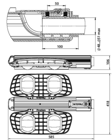
Рисунок 3. Габаритный чертеж
